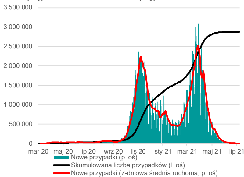
Dzienna liczba przeprowadzonych testów na koronawirusa oraz skumulowana liczba przypadków zakażeń koronawirusem
