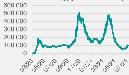
Odsetek pozytywnych testów (% , 7-dniowa średnia ruchoma)
